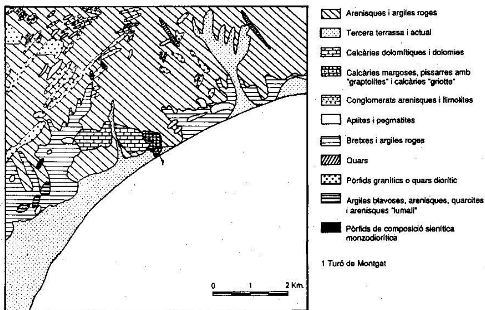
Fig. 2: Composició geològica d'el Maresme.
