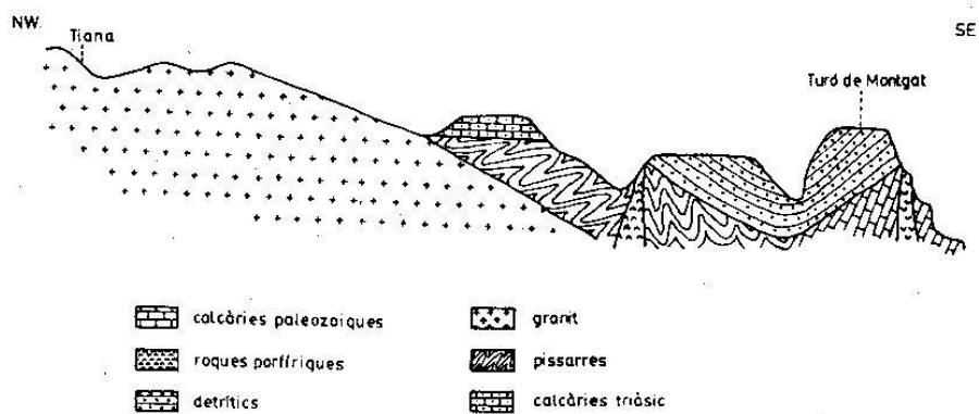
Fig. 3: Tall geològic del Turó de Montgat.
